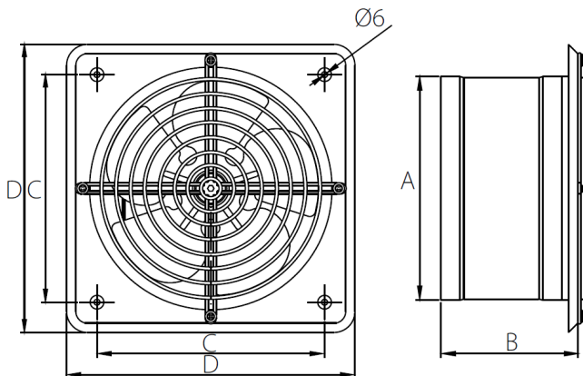
Wymiary wentylatora WB-S 200
